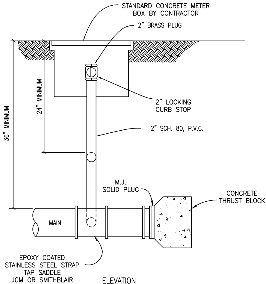
ELEVATION
